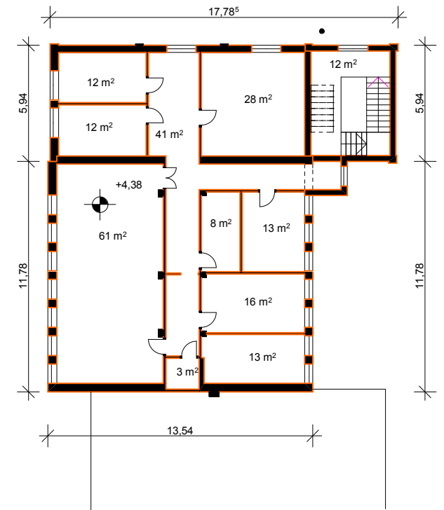
EMELETI ALAPRAJZ
