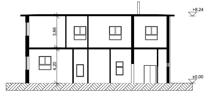
A-A METSZET
